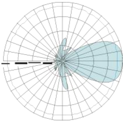
水平面波束宽度
