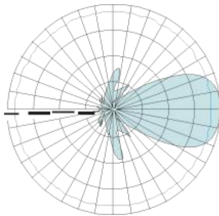
垂直面波束宽度
